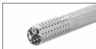
2 Spülkanäle / 2 irrigation channel
